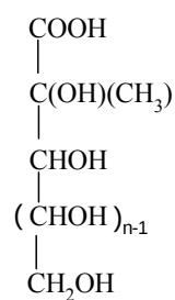
sacharinové kyseliny (2-methylaldonové kys.)
