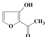
isomaltol
