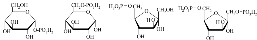
\alpha -D-Glc p -1-fosfat (Coriho ester)
