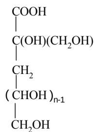
isosacharinové kyseliny (2-hydroxymethyl- 3-deoxyaldonové kys.)
