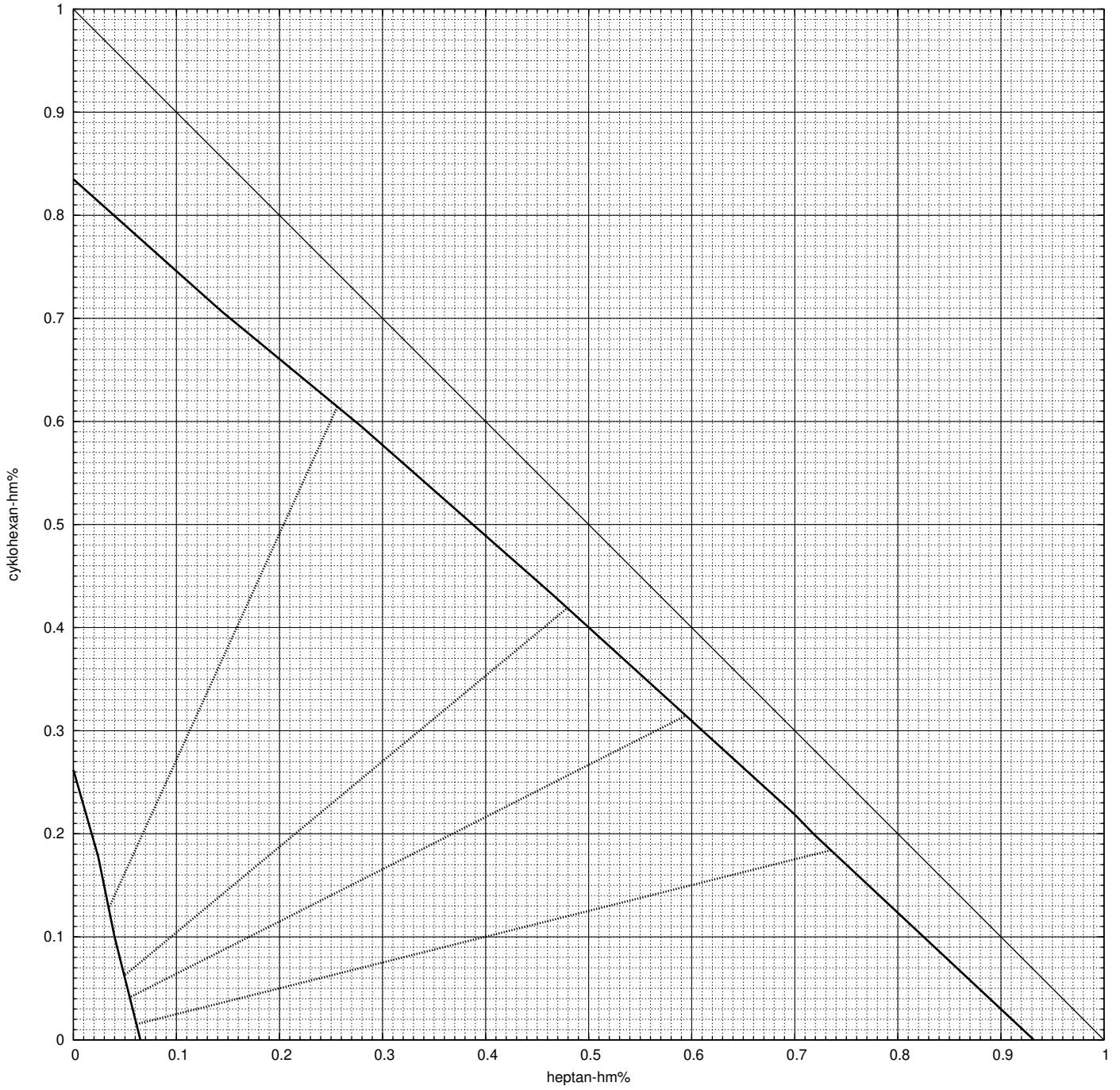
ANILIN-CYKLOHEXAN-HEPTAN (25 C)
