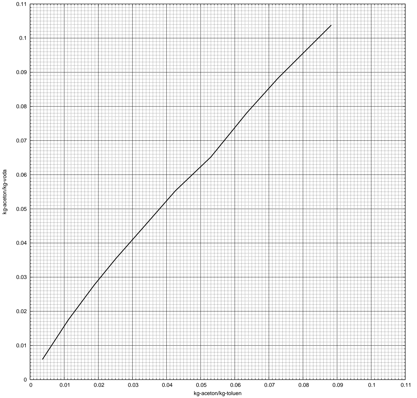
VODA-ACETON-TOLUEN (30C)
