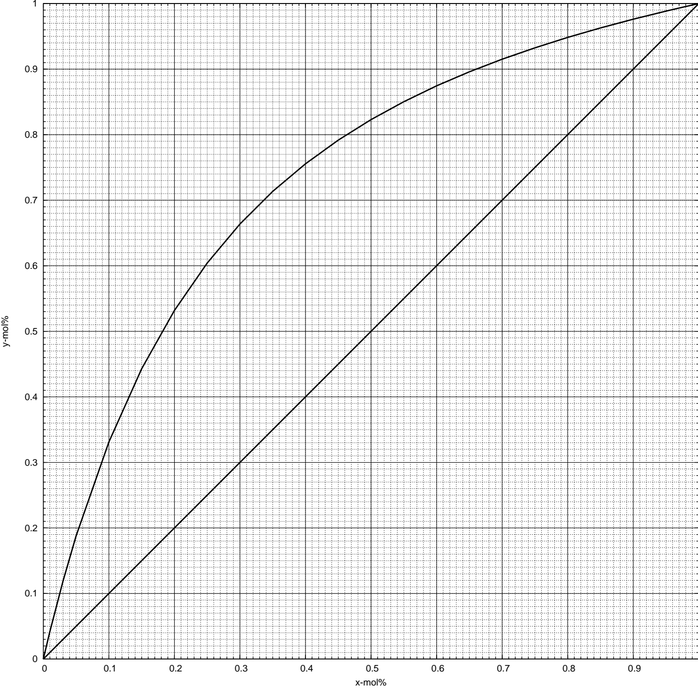
ETANOL-BUTANOL ( p=101.325 \text{ kPa} )
