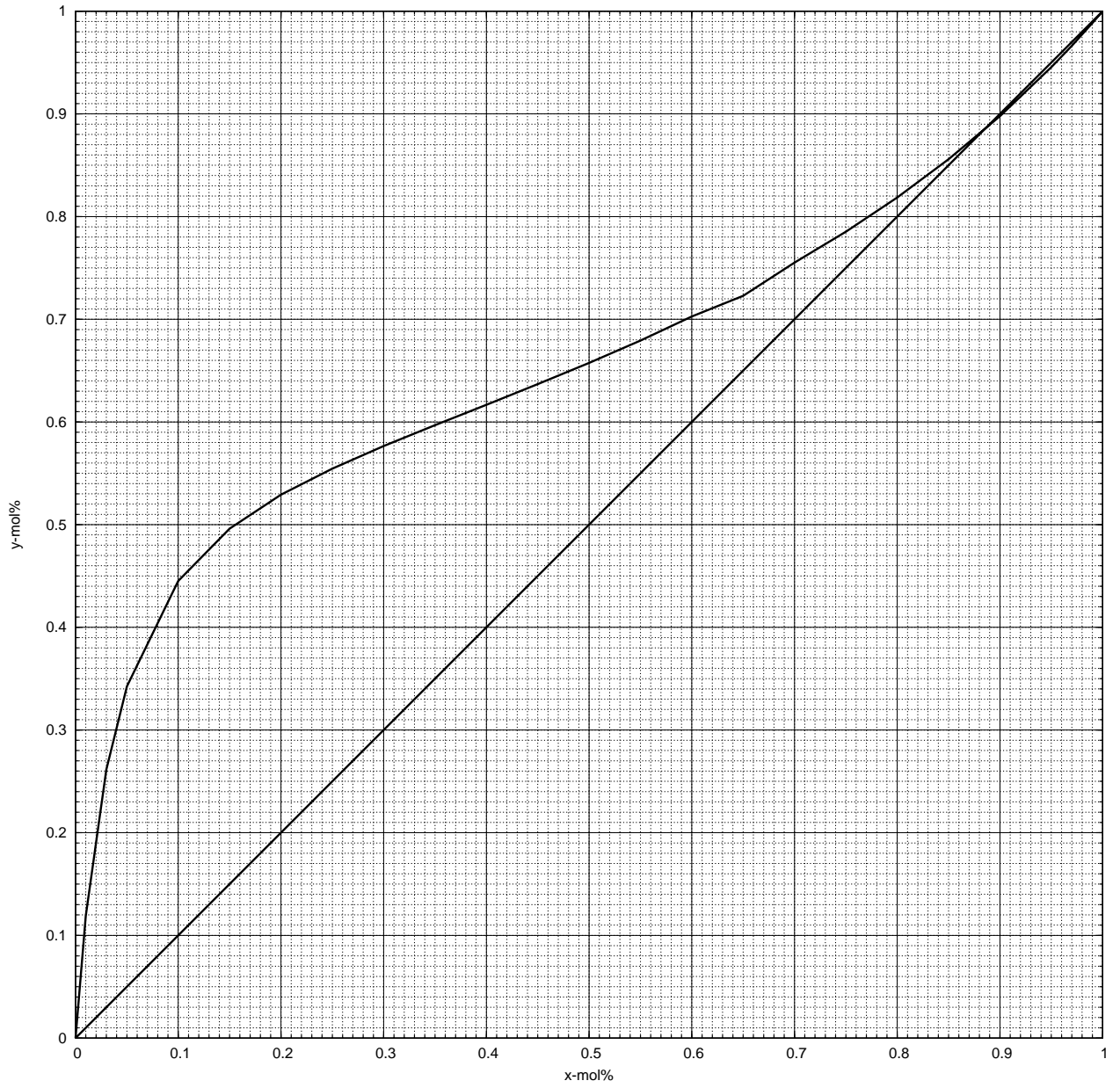
ETANOL-VODA (p=101.325 kPa)
